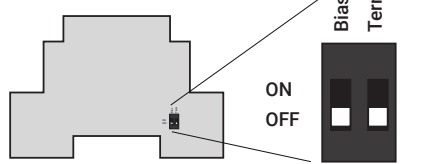
Abbildung 3: Die Bias-Spannung und der Terminierungswiderstand DIP-Schalter
